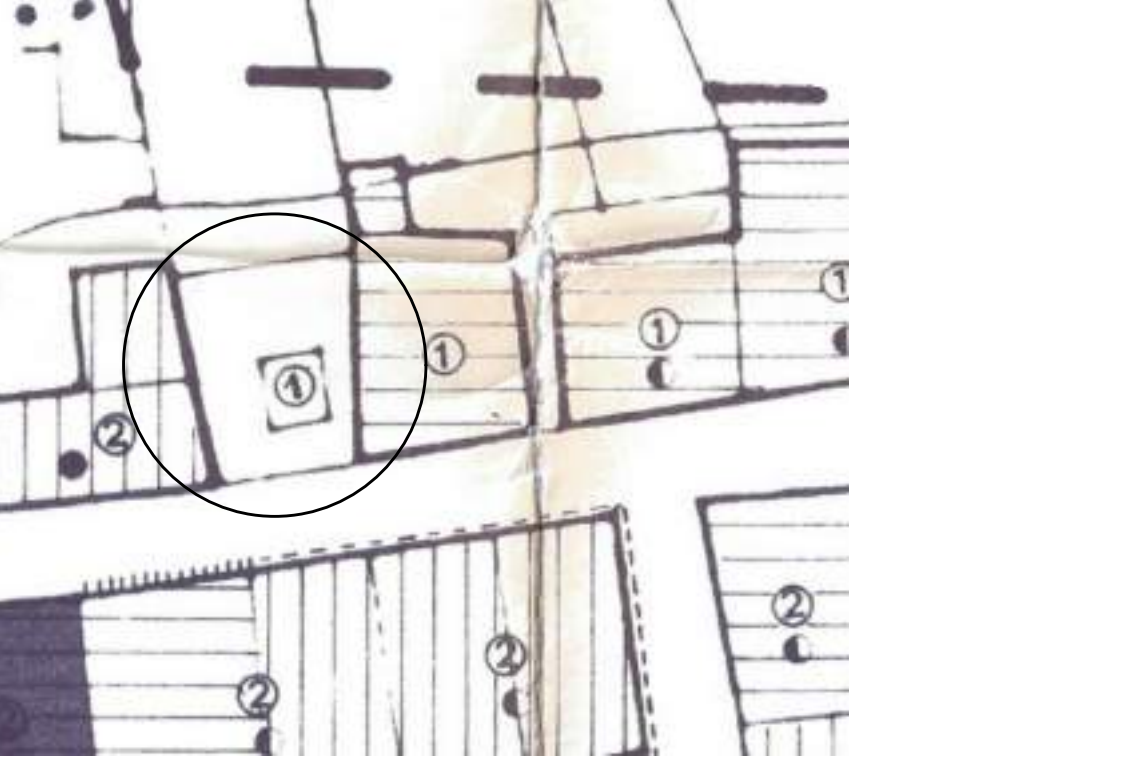
STRALCIO DI P.P. TAVOLA 5 scala 1:500
