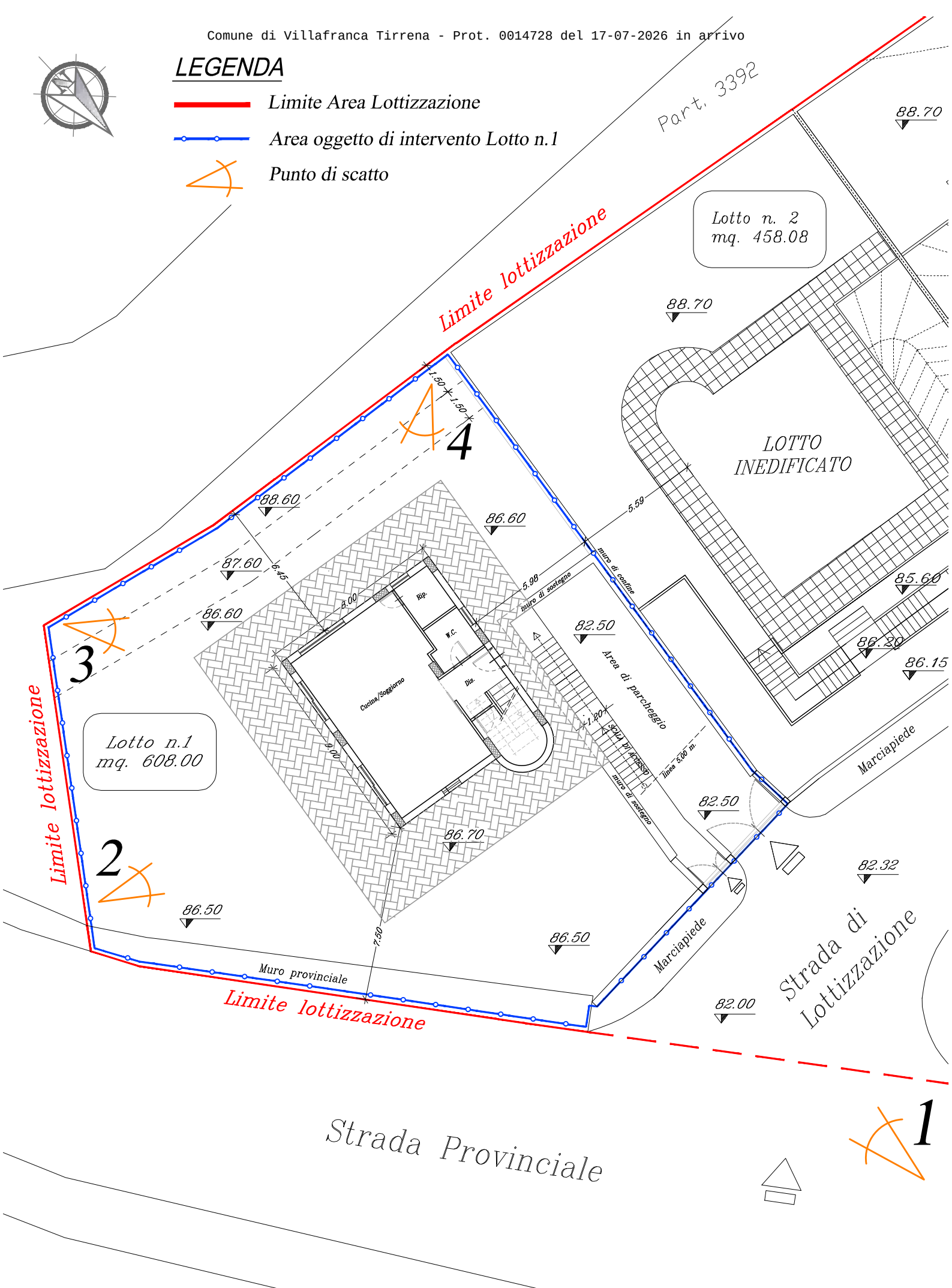
Planimetria con indicazione dei punti di scatto - Scala 1:200
